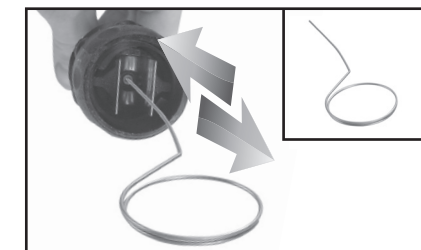
Nadel zur Reinigung der Düse, Abb. 13
