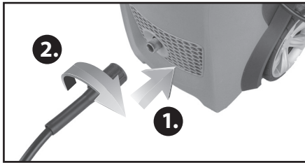
Anschluss des Druckschlauches an den Austritt des Druckwassers, Abb. 5
