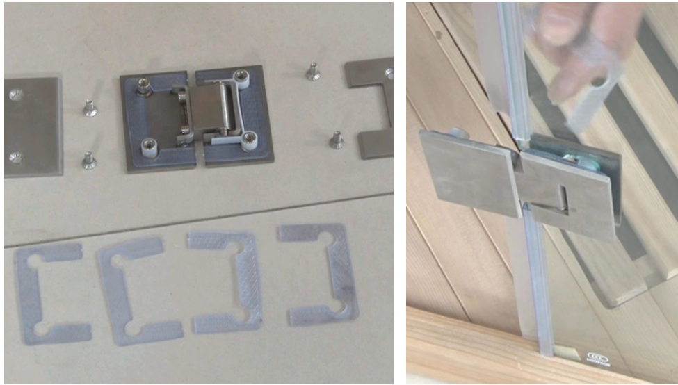
6. umístěte skleněná dvířka
