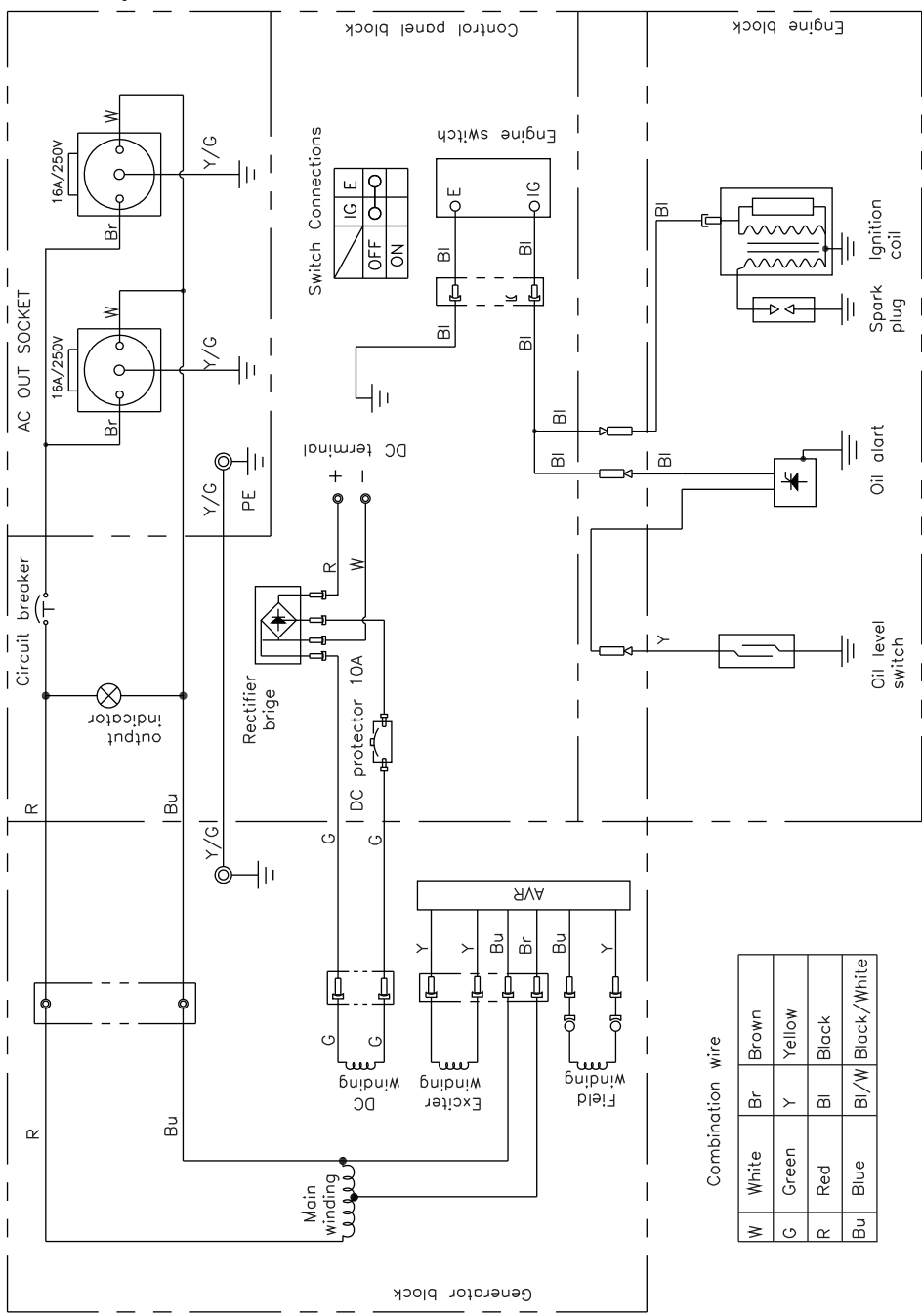
Stromlaufplan 1 2500-C/3000-C/3500-C
