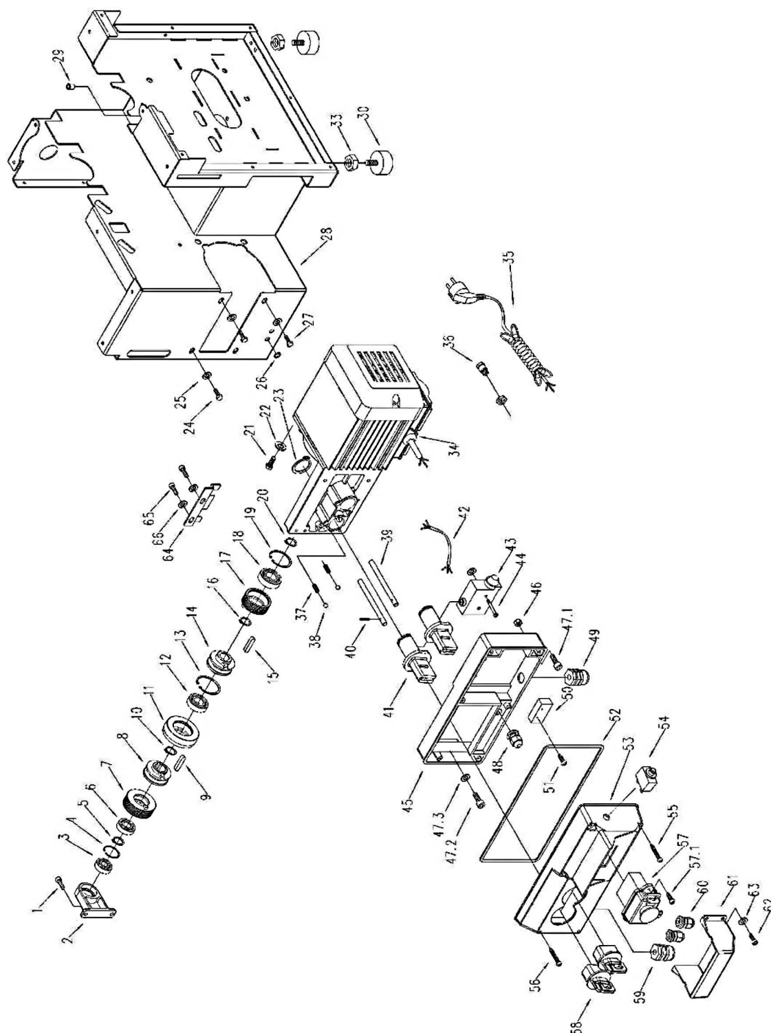
Obr. 49: Rozpadové schéma 1
