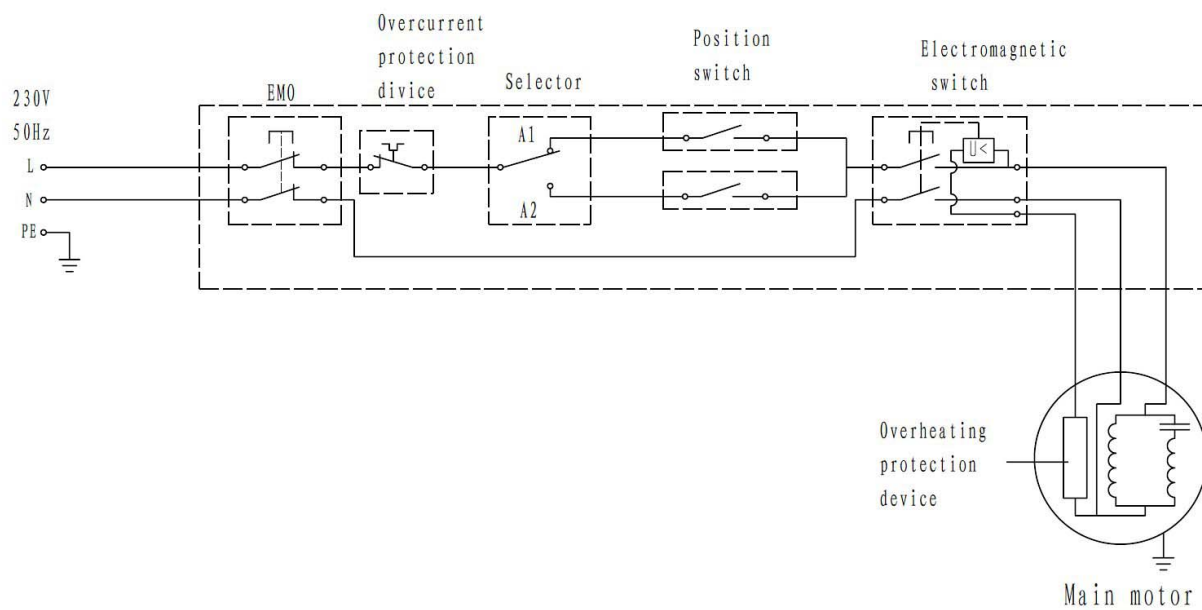
Obr. 54: Schéma zapojení
