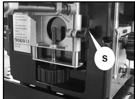
Obr. 41: Nastavení výšky stolu
