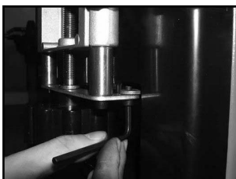
Obr. 11: Montáž frézovacího stolu na pracovní stůl
