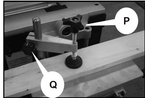
Obr. 40: Zajištění obrobku pomocí upínacího zařízení
