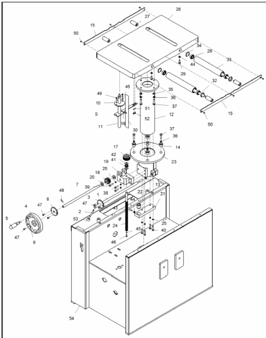
FS41N.10.00.00 DICKENTISCH - HÖCHENVERSTELLUNG
