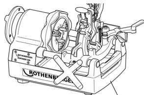
Vis de vidange d'huile
