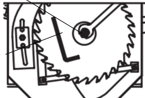
Imbus klíč
