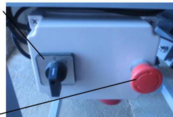
Hlavní vypínač 0 - 1
