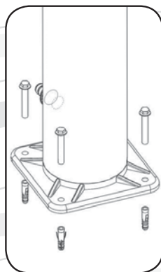
Obrázek 1 – Kotvení sprchy
