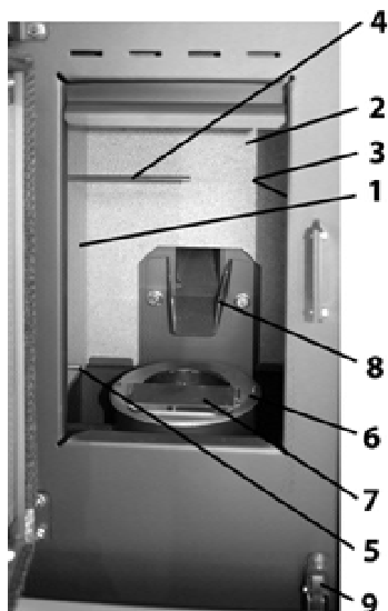
Obrázek 17: Prostor topeniště
