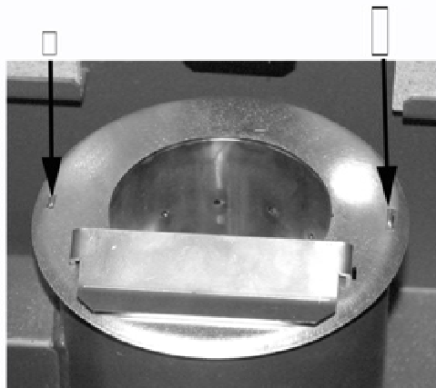
Obrázek 11: Správně nasazený hořák pelet
