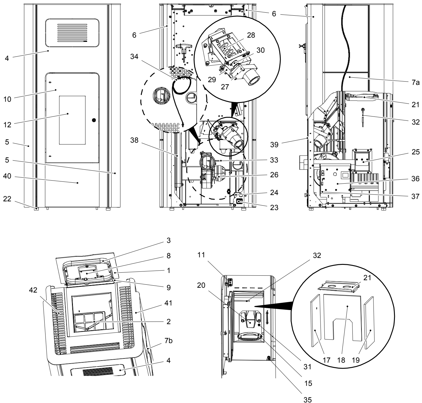
Obrázky 27: Náhradní díly ALMERIA 32-C
