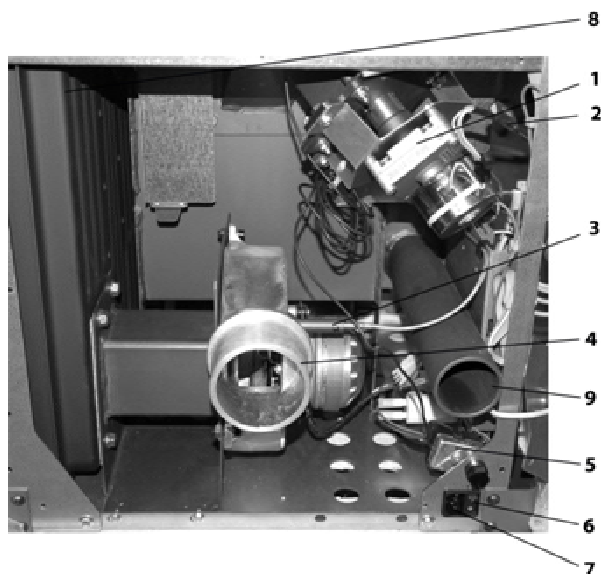
Obrázek 10: Šnekový motor
